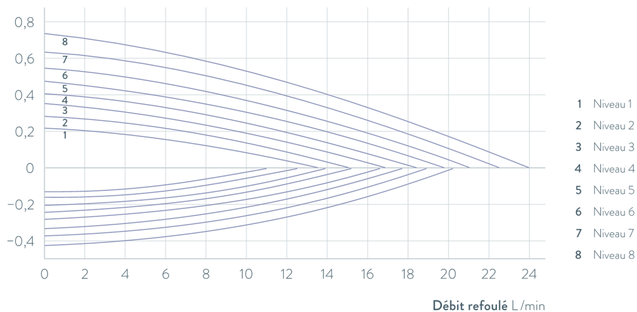
Fig. 95: Caractéristique de la pompe Universa MAX avec pompe refoulante-aspirante (pompe Varioflex)
