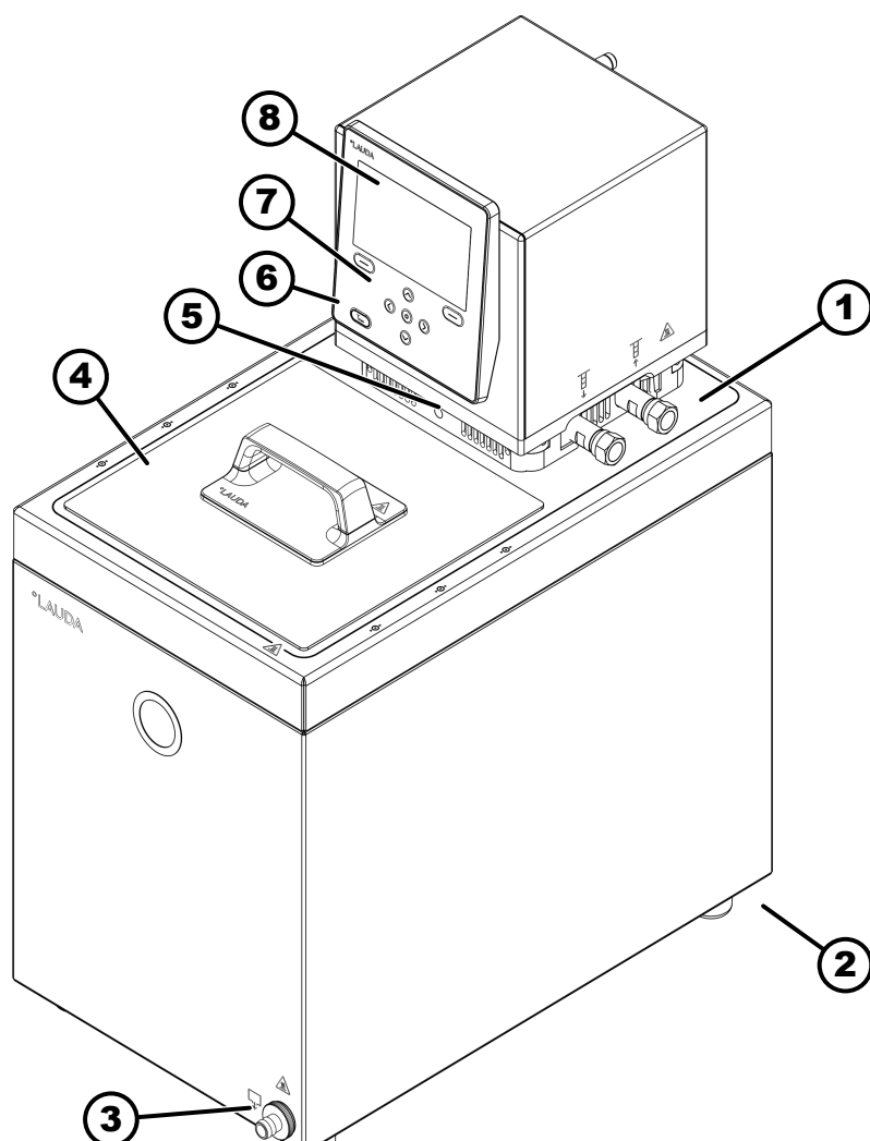
Fig. 5: Thermostat chauffant MAX, vue frontale
