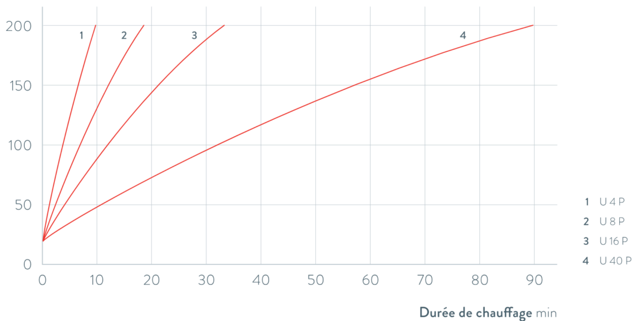
Fig. 89: Courbes de montée en température pour thermostats chauffants Universa PRO
