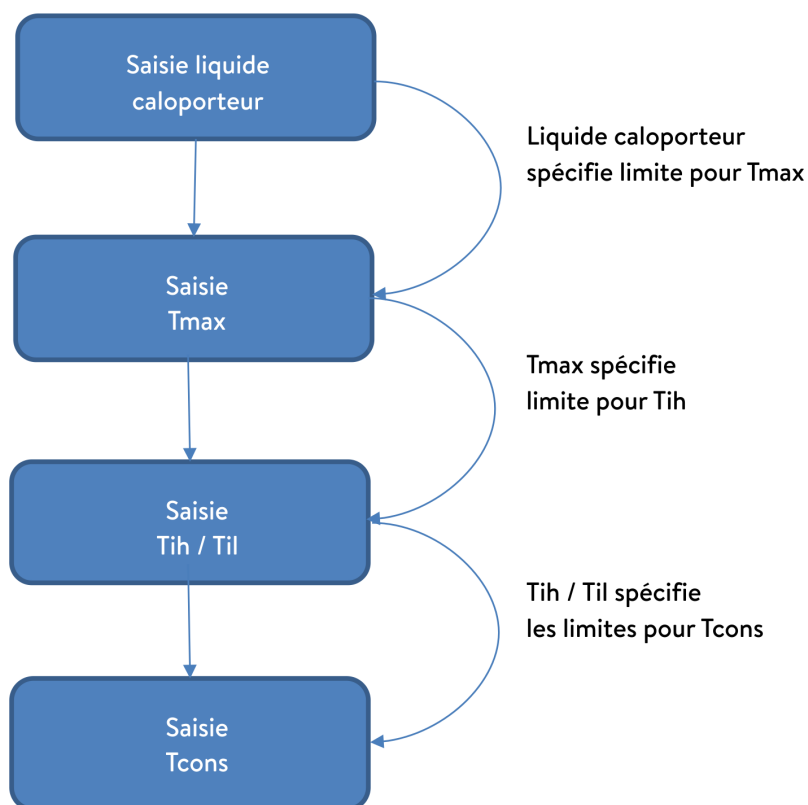
Fig. 44: Ordre chronologique des saisies
