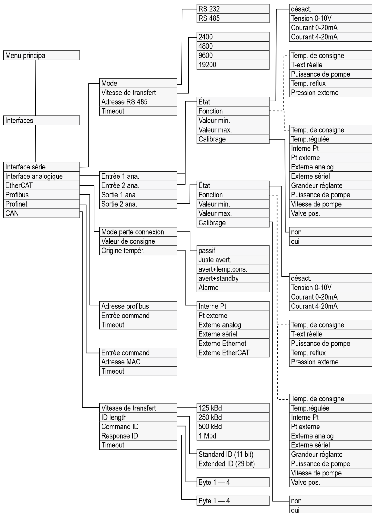
Fig. 66: Structure du menu partie 4, pour MAX et PRO
