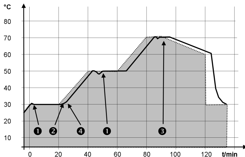
Fig. 82: Déroulement du programme température de consigne et température réelle
