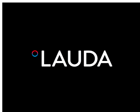
Fig. 42: Écran d'accueil
