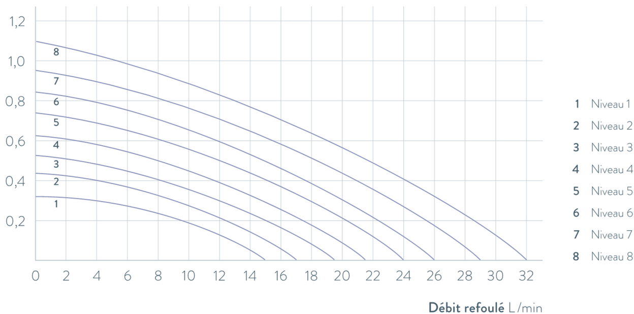
Fig. 94: Caractéristique de la pompe Universa MAX avec pompe de refoulement (pompe Vario) pour une profondeur du bain de 320 mm
