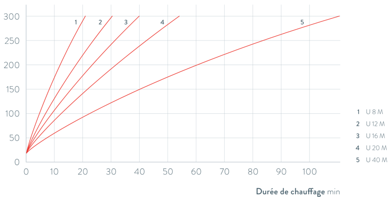
Fig. 90: Courbes de montée en température pour thermostats chauffants Universa MAX
