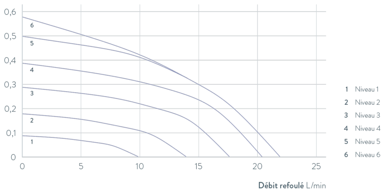
Fig. 93: Caractéristique de la pompe Universa PRO
