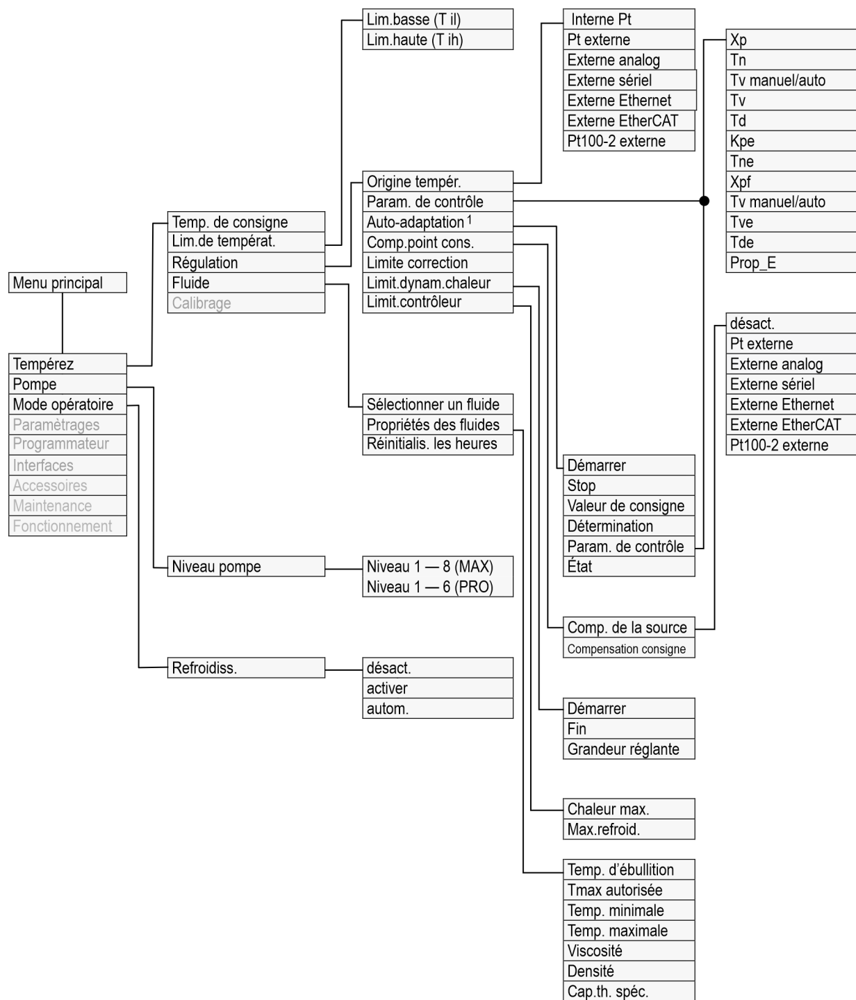
Fig. 63: Structure du menu partie 1, pour MAX et PRO
