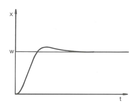
Fig. 70: Paramètre de régulation X_p trop élevé
