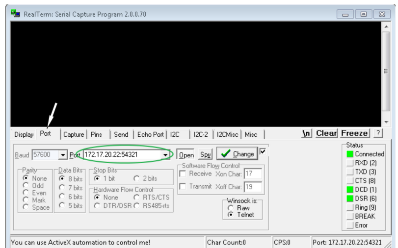
Fig. 58: Saisie dans le champ Port
