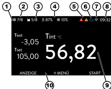
Fig. 39: Fenêtre de base avec barre d'état, affichage de la température et barre des touches programmables
