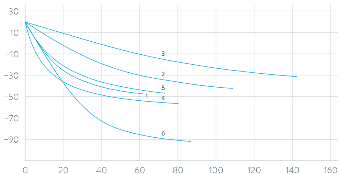
Fig. 92: Courbes de refroidissement pour cryothermostats Universa MAX
