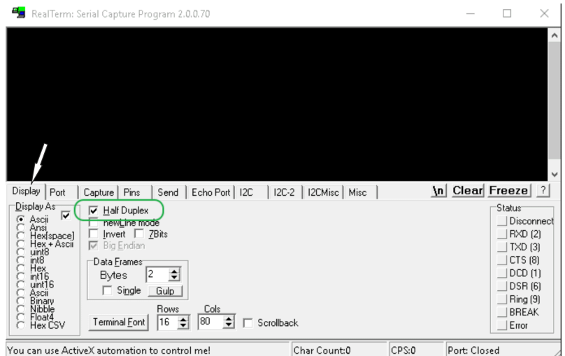
Fig. 57: Programme « RealTerm »
