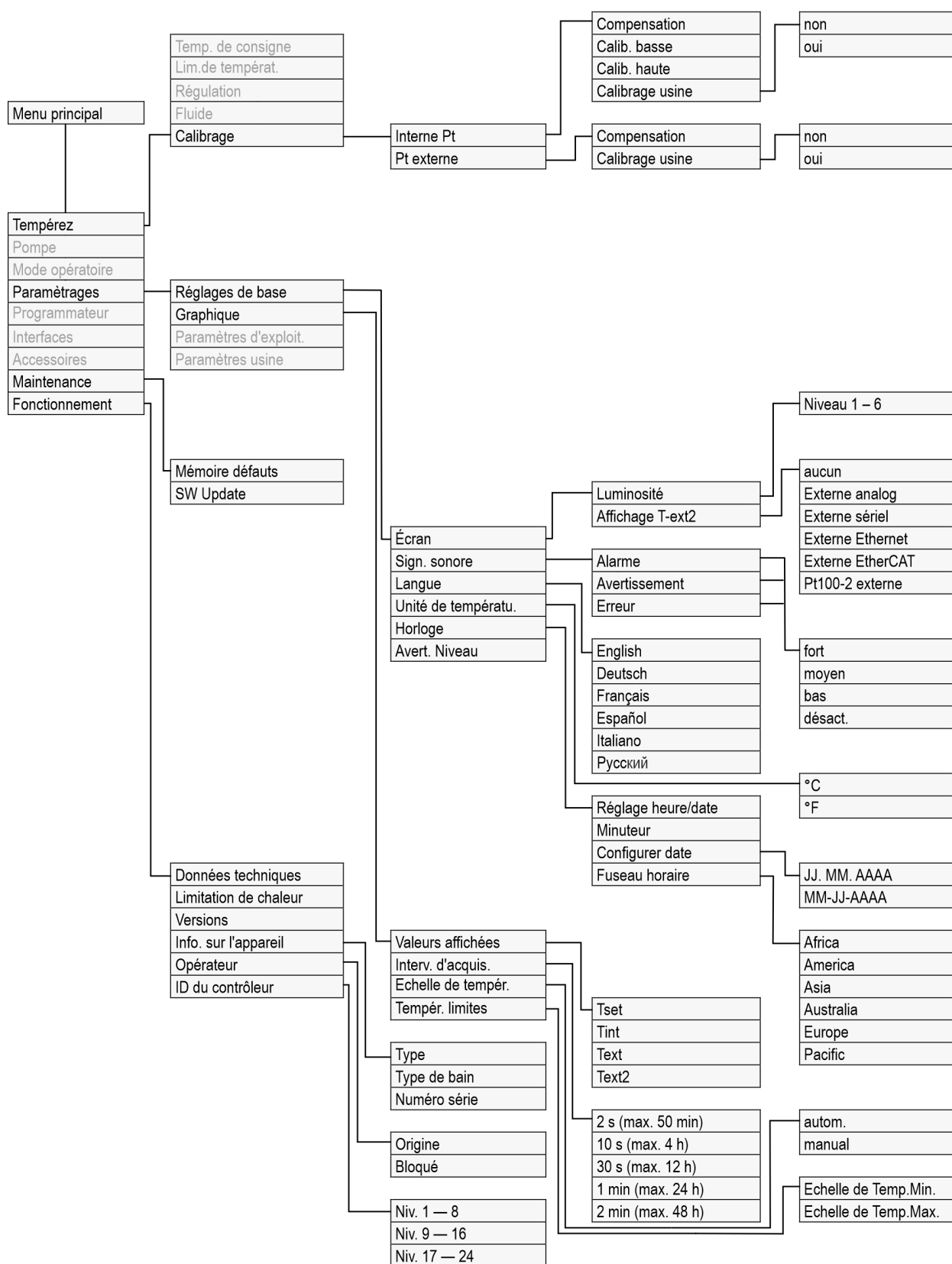
Fig. 64: Structure du menu partie 2, pour MAX et PRO
