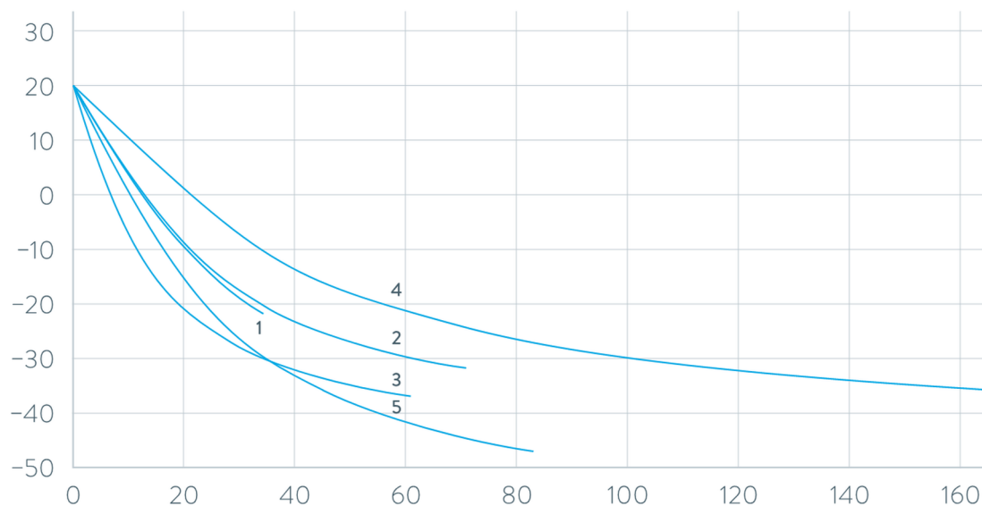
Fig. 91: Courbes de refroidissement pour cryothermostats Universa PRO
