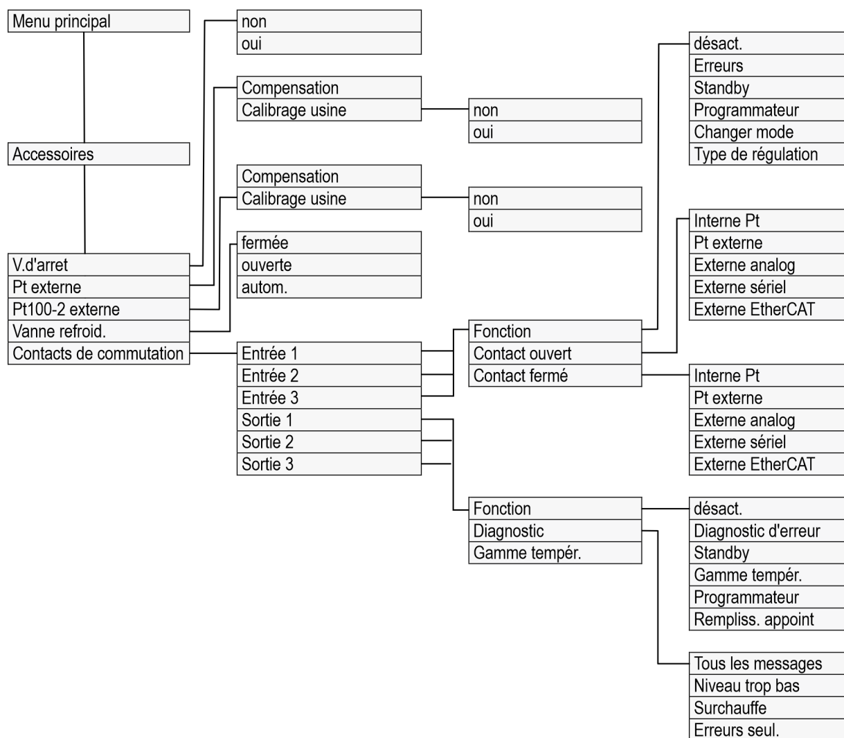
Fig. 67: Structure du menu partie 5, pour MAX et PRO
