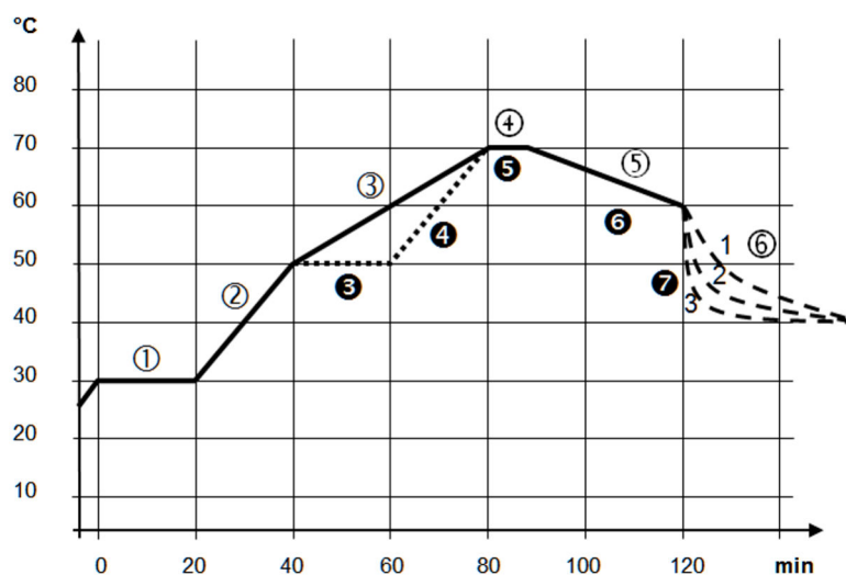
Fig. 81: Déroulement du programme (avant et après), exemple
