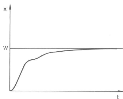
Fig. 73: Paramètres de régulation T_n et T_v trop grands
