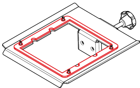
Fig. 33: Joint plat sur l'unité de bains/ l'adaptateur de bain
